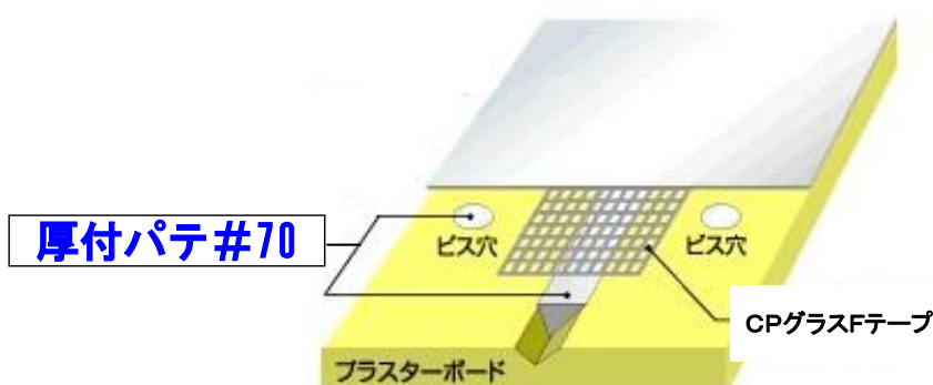
プラスターボードの施工イメージ
